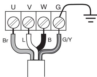
Diagrama de cableado
